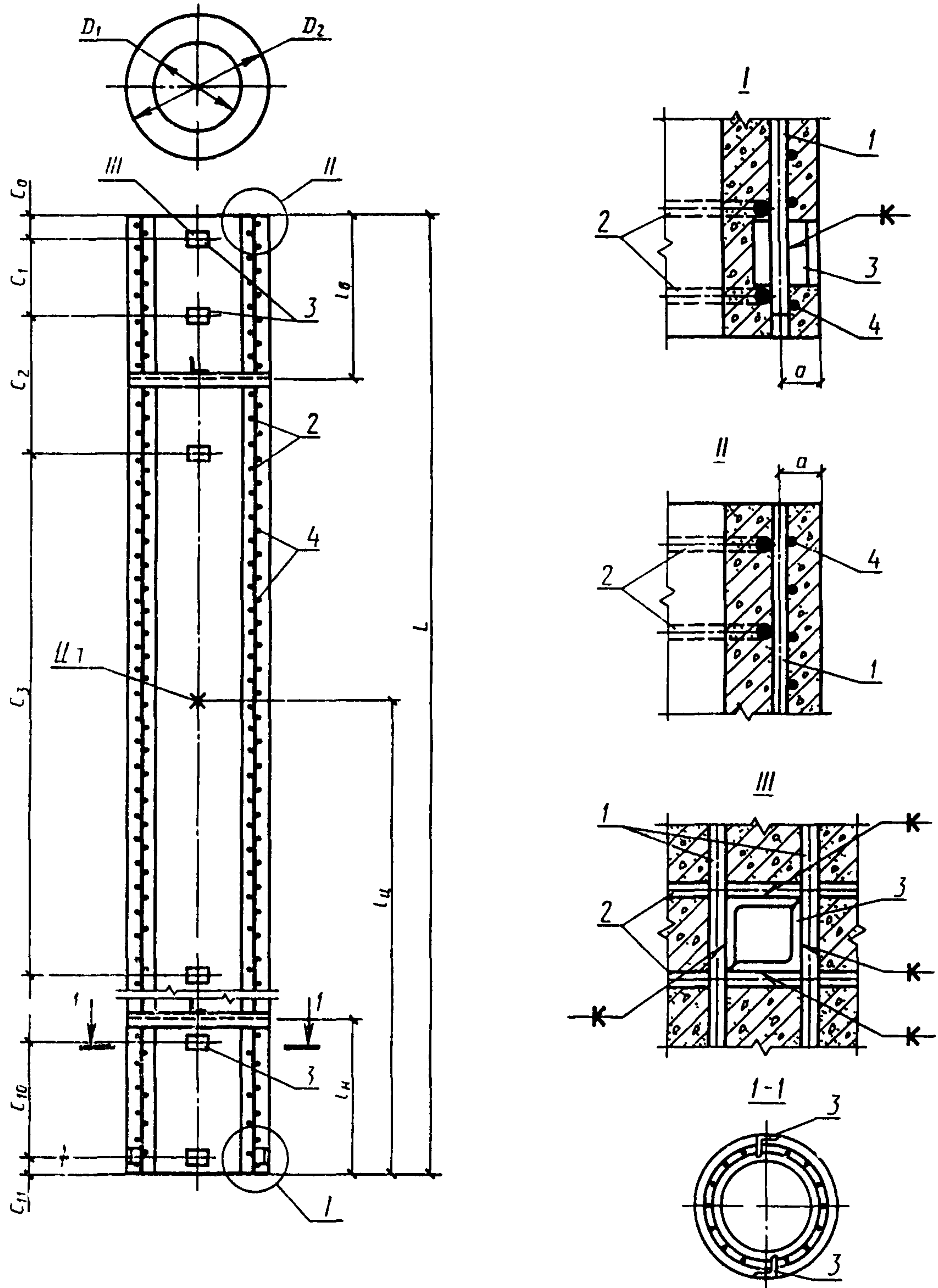
1 — продольная арматура 2 — монтажные кольца 3 — закладные изделия 4 — спираль, a — расстояние от наружной поверхности стойки до оси продольной арматуры, C_0 - C_2 C_{10} - C_{11} — привязка закладных изделий \tau — центр тяжести L — длина стойки l_{II} — расстояние до центра тяжести l_{III} , l_{IV} — расстояния до мест установки диафрагм D_1 — внутренний диаметр стойки D_2 — наружный диаметр стойки
